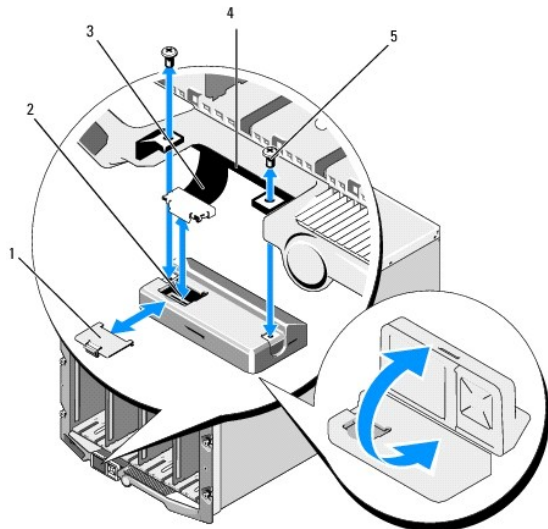
図 C-1. LCD モジュールの取り外しと取り付け
